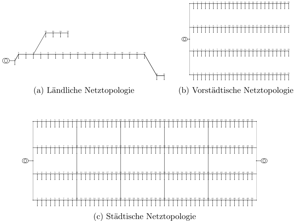
Abbildung 4.2: Untersuchte elektrische Niederspannungsternetztopologien
