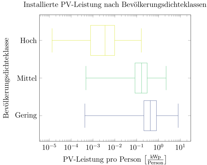
Abbildung 4.3: Installierte Photovoltaik (PV)-Leistung in kWp pro Person auf Gebäuden in Niederspannungsnetzen (Daten aus [14]), differenziert nach Postleitzahl (PLZ)-scharfen Bevölkerungsdichteklassen aus [13].
