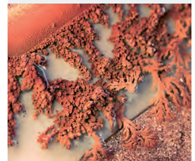
Korrosionsschutz für leistungselektronische Module. © Fraunhofer IISB » Seite 12
