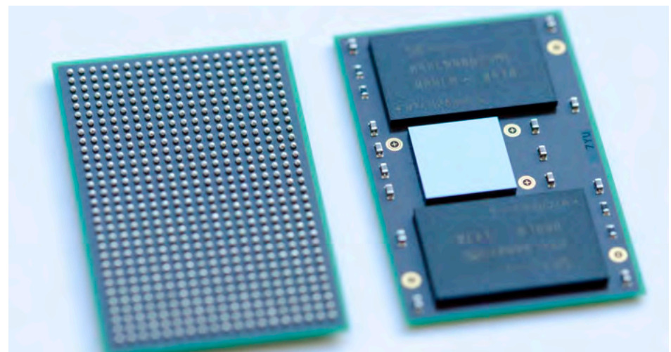
Fine-Pitch-Package-Substrat für ein multifunktionales System-on-Chip. © Fraunhofer IIS / EAS
