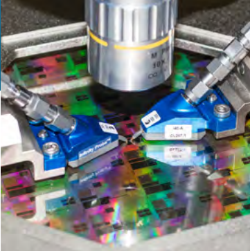
Charakterisierung eines Wafers mit Komponenten in LF15A-Technologie.
