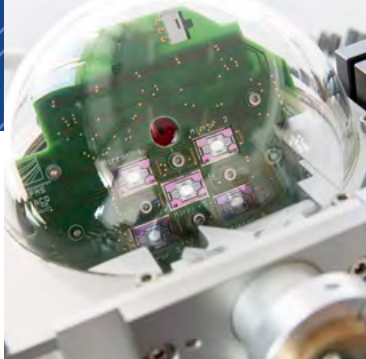
Innerhalb der FMD gibt es für jede einzelne Komponente eines LiDAR-Systems vielfältige FuE-Aktivitäten. © Fraunhofer IPMS
