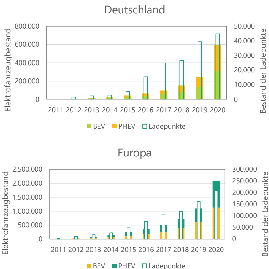
Abbildung 2: Bestand von Elektrofahrzeugen unterschieden nach BEV und PHEV, sowie Ladepunkte in Deutschland und Europa 2011 bis 2020. Daten von (EAFO 2021)
