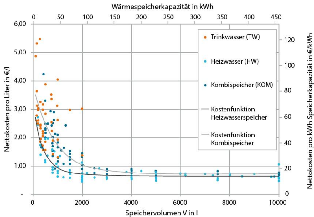
Abb. 2-14: Spezifische Wärmespeicherkosten (nach Samweber et al. 2017)
