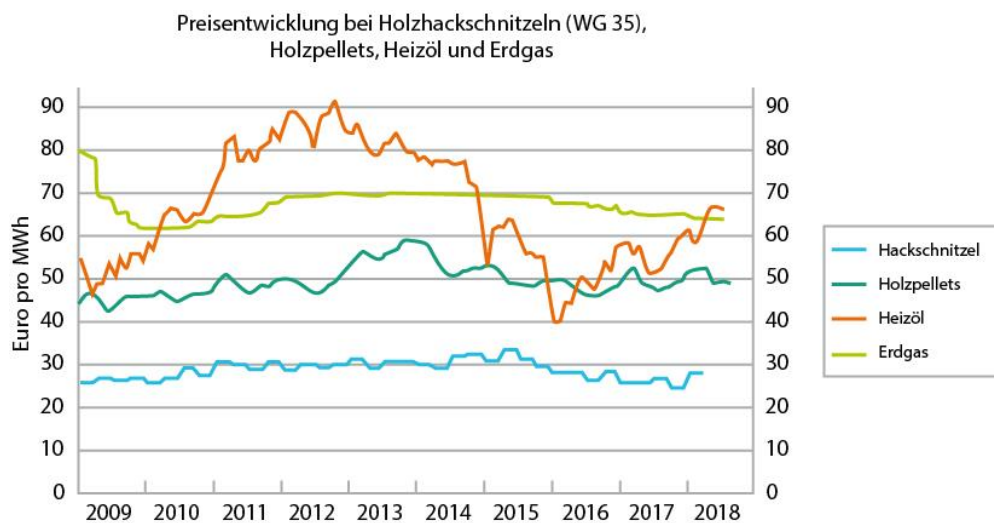
Abb. 2-13: Preisentwicklung bei Holzackschnitzeln, Holzpellets, Heizöl und Erdgas 2009 bis 2018 (MwSt inklusive) (nach C.A.R.M.E.N. 2018)
