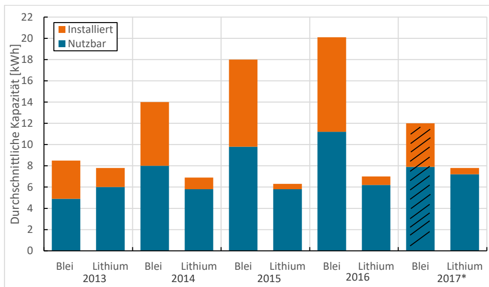
Abb. 2-16: Entwicklung der durchschnittlichen Speicherkapazitäten von Solarstromspeichern von Mai 2013 bis April 2017. *) Die Anzahl an Bleispeichern im laufenden Jahr 2017 wird mit 11 Systemen als nicht repräsentativ eingestuft (nach Figgenger et al. 2017)
