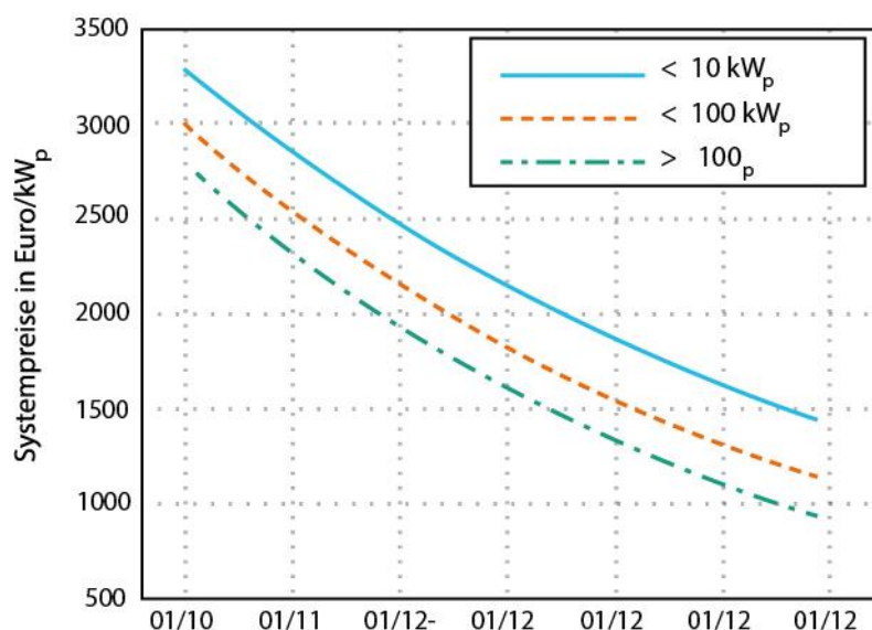
Abb. 2-2: Preisentwicklung der durchschnittlichen Systempreise für netzgekoppelte Photovoltaikanlagen (nach Wesselak et al. 2016, S. 105)
