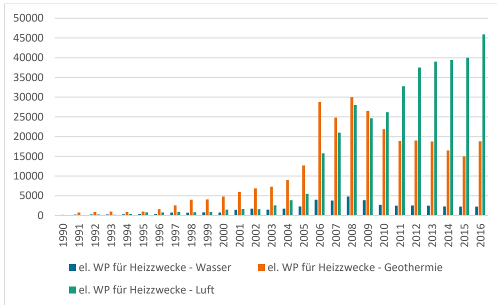
Abb. 2-6: Absatzzahlen von elektrischen Heizwärmepumpen nach Art der Wärmepumpe in Deutschland (nach Born et al. 2017)
