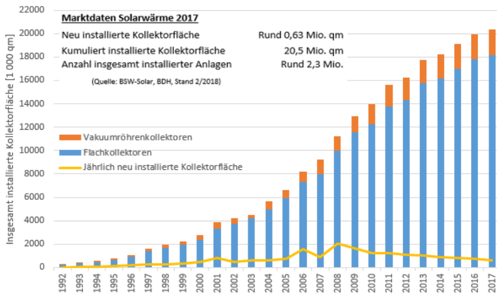
Abb. 2-5: Zubau an Solarwärmesystemen in Deutschland (gerundete Werte, Abbau von Altanlagen nicht berücksichtigt) (nach BSW-Solar 2018)
