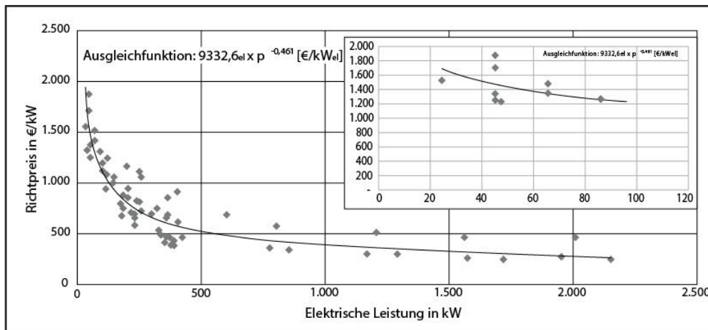
Abb. 2-10: Preise für Erdgas BHKW ohne gesetzliche Mehrwertsteuer (Datenquelle: ASUE 2016)
