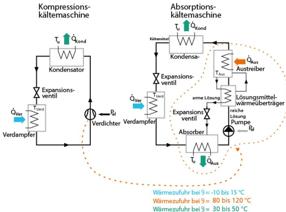
Abb. 2-15: Aufbau einer Kompressionskälte- (links) und einer Absorptionskältemaschine (rechts) (nach ITW 2013)
