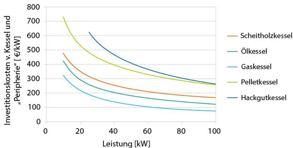
Abb. 2-12: Spezifische Investitionskosten von Heizkessel bis 100 kW inkl. Peripherie (Bezugszeitraum: 2000 bis 2010) (nach Kalt et al. 2009)
