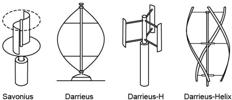
Abb. 2-4: Rotortypen vertikaler Windkraftanlagen (nach Schmelter et al. 2015)
