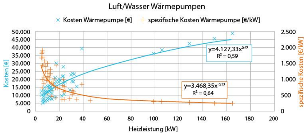
Abb. 2-7: Kostenkurve der Luft-Wasser-Wärmepumpe (nach Wolf et al. 2014)
