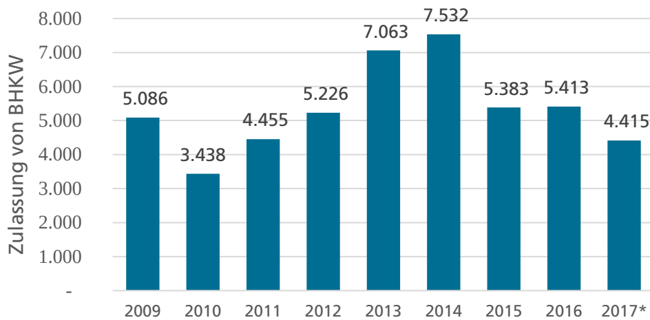
Abb. 2-8: Zulassung von BHKW-Anlagen in Deutschland in den Jahren 2009 bis 2017 (* Zulassungsanträge für 2017 sind in der Datenquelle noch nicht vollständig berücksichtigt) (Datenquelle: BAFA 2018)
