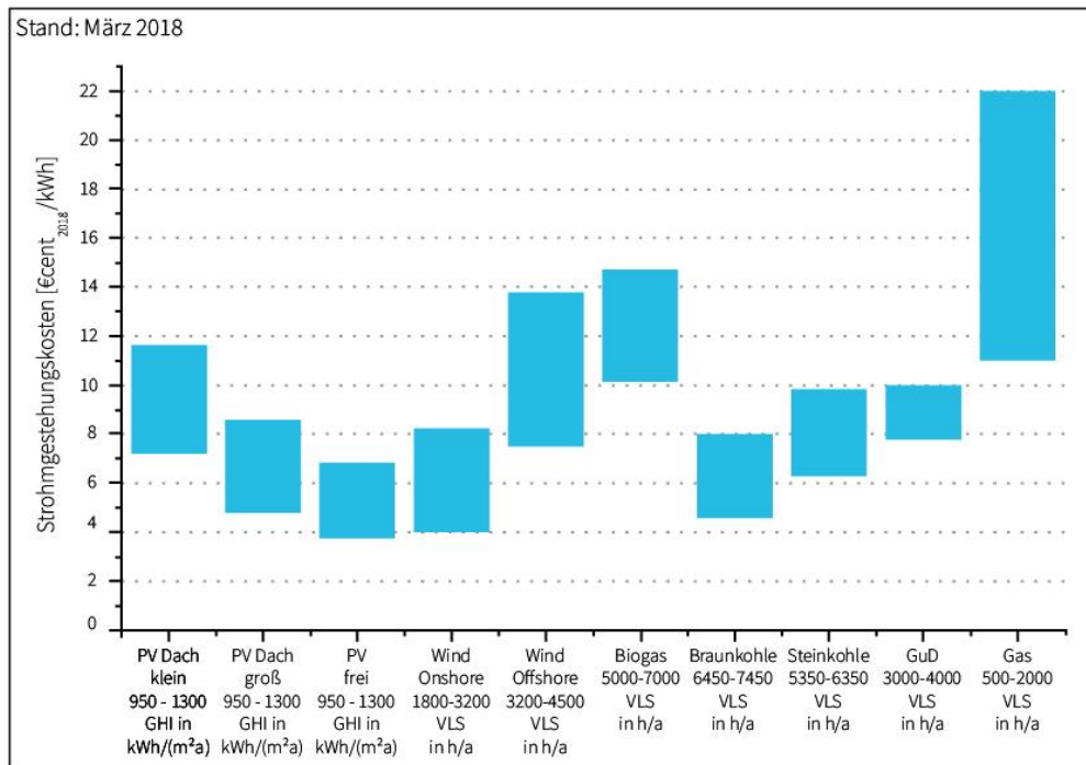
Abb. 2-3: Stromgestehungskosten für erneuerbare Energien und konventionelle Kraftwerke an Standorten in Deutschland im Jahr 2018 (nach Kost et al. 2018)
