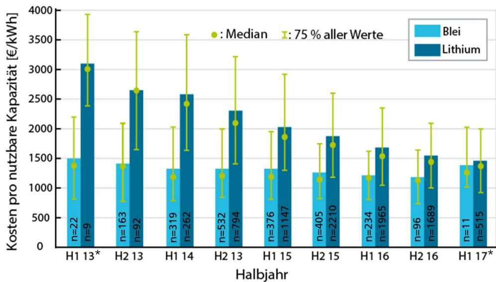
Abb. 2-18: Entwicklung der durchschnittlichen Endverbraucherpreise von Solarstromspeichern von Mai 2013 bis April 2017 pro nutzbare Kilowattstunde (* Die Anzahl aller Systeme in H1 13 und diejenigen der Blei-Systeme in H1 17 wird als nicht repräsentativ eingestuft.) (nach Figgner et al. 2017)
