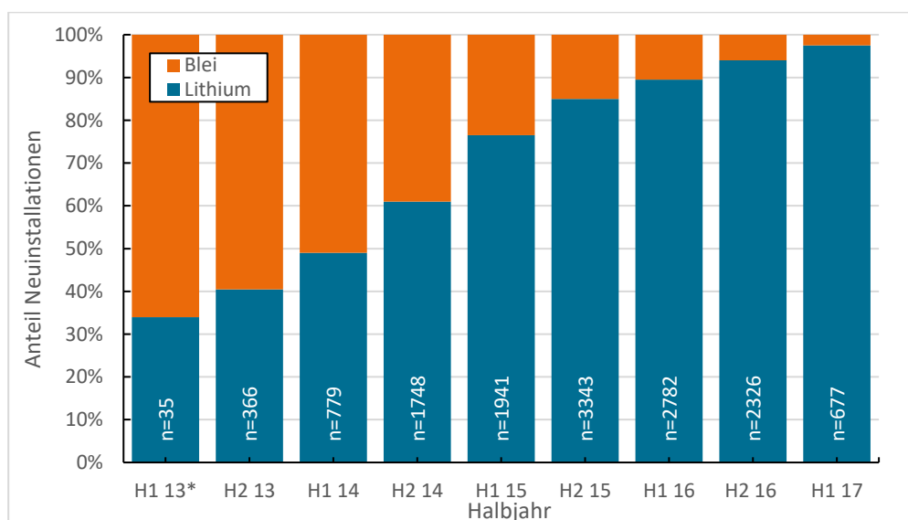
Abb. 2-17: Anteil der Batterietechnologien der beim Speichermonitoring registrierten PV-Speicher nach Anzahl von Mai 2013 bis April 2017 (nach Figgener et al. 2017)
