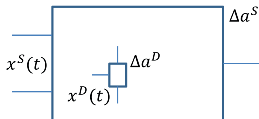
Abbildung 4.33: Übergang von Bauelemente- zu Schaltungsdegradation
