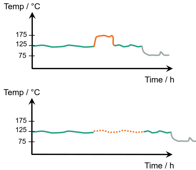
Abbildung 4.20: Umrechnung auf einheitliche Temperatur im Mission Profile
