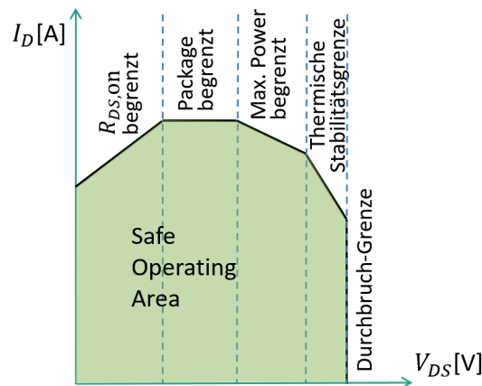
Abbildung 4.7: Betriebsgrenzen eines Leistungs-MOSFETs [153]
