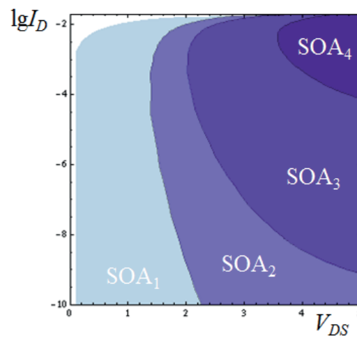
Abbildung 4.12: SOA-Diagramm abgeleitet aus Bild 4.11 [77]
