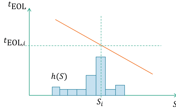
Abbildung 4.18: Lastverteilung im Belastbarkeitsdiagramm
