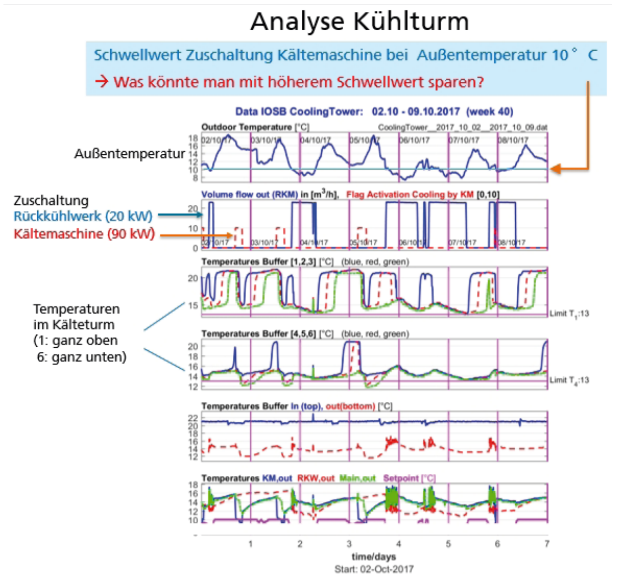
Abbildung 22: Messdaten eines Kühlturmes von einer Woche (2.-9.10.2017). Bei Außentemperatur größer 10°C wird statt des Rückkühlwerkes die Kältemaschine aktiviert – hier könnte ein höherer Wert (z.B. T_a=18^\circ\text{C} ) viel Energie einsparen.
