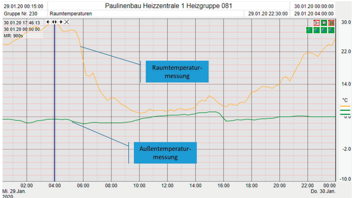
Abbildung 17: Vergleich der Außentemperatur- zur Raumtemperaturmessung
