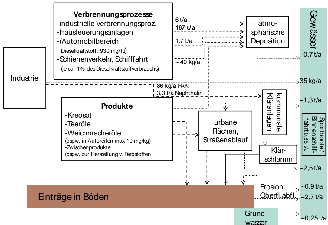
Abbildung 6: Qualitative PAK Stoffströme in Verbindung mit Gewässereinträgen pro Jahr, Deutschland 2010-2013
