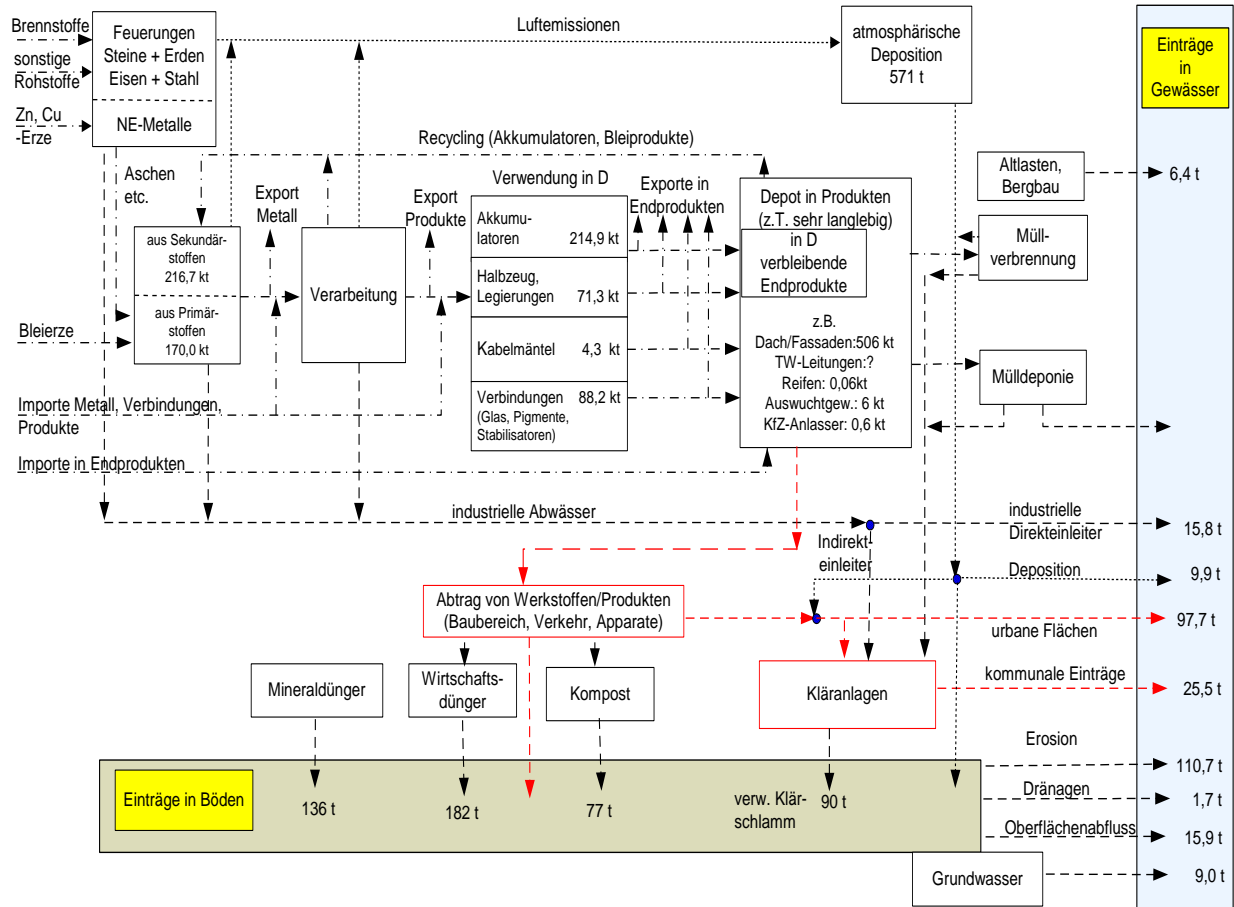
Abbildung 7: Bleiproduktion und -verwendung und qualitative Stoffströme in Verbindung mit Gewässereinträgen, Deutschland 2000 (Hillenbrand et al., 2007)
