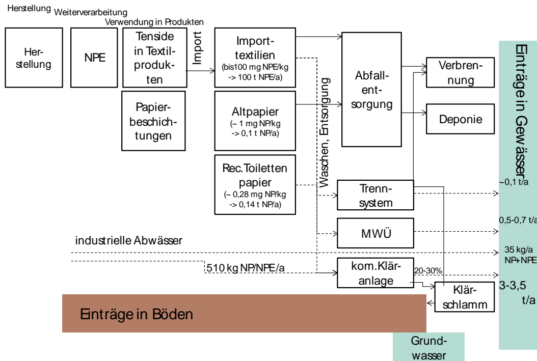
Abbildung 2: Qualitative Nonylphenol Stoffströme in Verbindung mit Gewässereinträgen pro Jahr für den Zeitraum 2010-2013 in Deutschland
