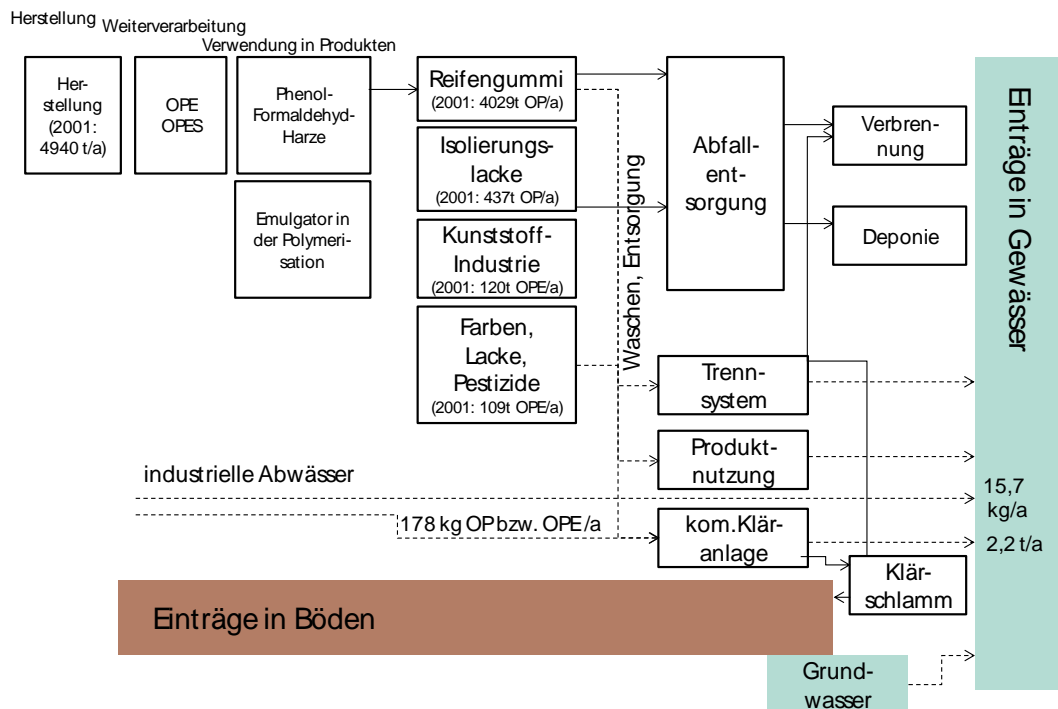
Abbildung 4: Qualitative Octylphenol Stoffströme in Verbindung mit Gewässereinträgen pro Jahr für den Zeitraum 2010-2013 in Deutschland
