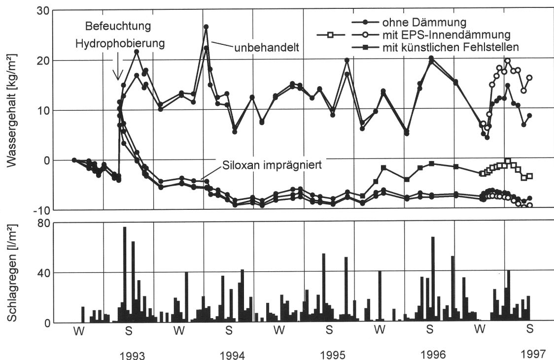
Bild 4: Gemessene Feuchteverläufe von exponierten Außenwandelementen aus Vollziegel-Sichtmauerwerk mit Angabe der Schlagregenbelastung in Dekadensummen.
