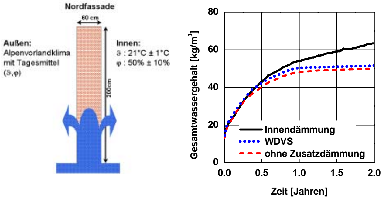
Bild 5: Zweidimensionale Berechnung der kapillaren Wasseraufnahme von Ziegelmauerwerk mit und ohne Dämmung unter natürlichen Klimabedingungen [6]
