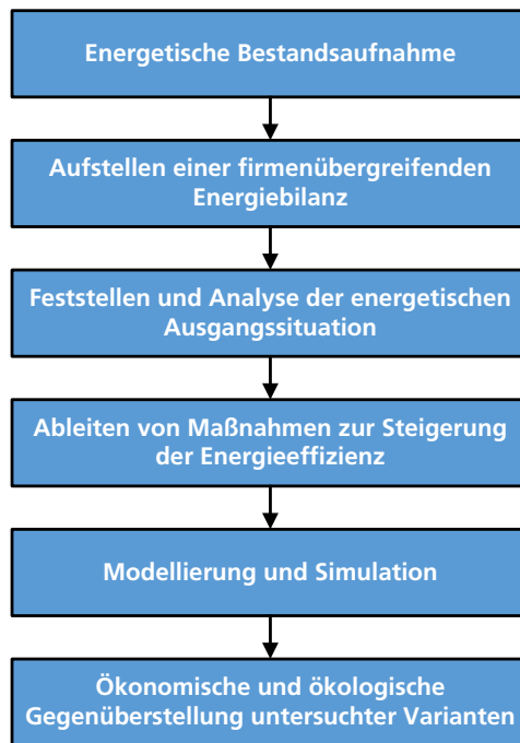
Abb. 1: Methodisches Vorgehen
