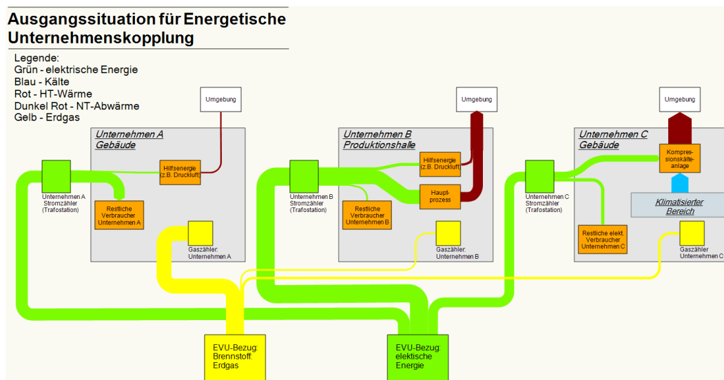
Abb. 2: Sankey-Diagramm der energetischen Ausgangssituation
