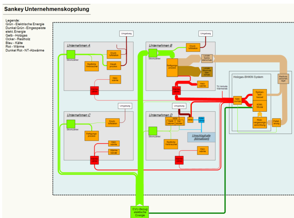
Abb. 3: Sankey-Diagramm Unternehmenskopplung mittels Holzgas-BHKW-System
