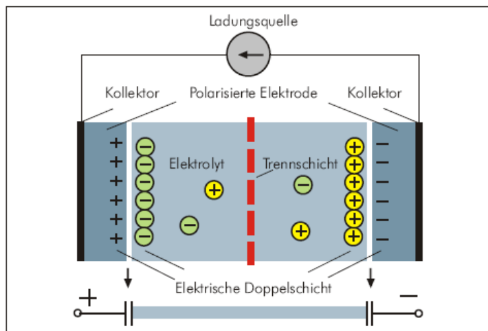
Abbildung 4-11: Funktionsprinzip eines elektrischen Doppelschicht-Kondensators
