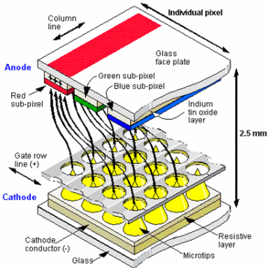
Abbildung 4-20: Schematischer Aufbau eine Field Emitter Displays
