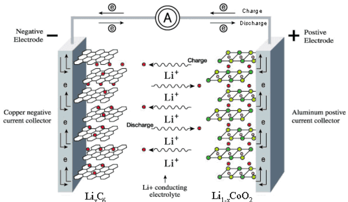
Abbildung 4-46: Funktionsprinzip des Lithium-Ionen-Systems
