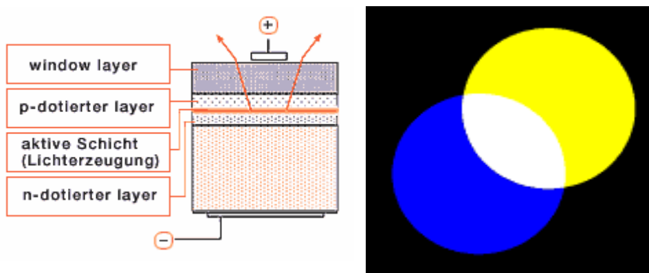
Abbildung 4-23: Funktionsweise einer Light Emitting Diode
