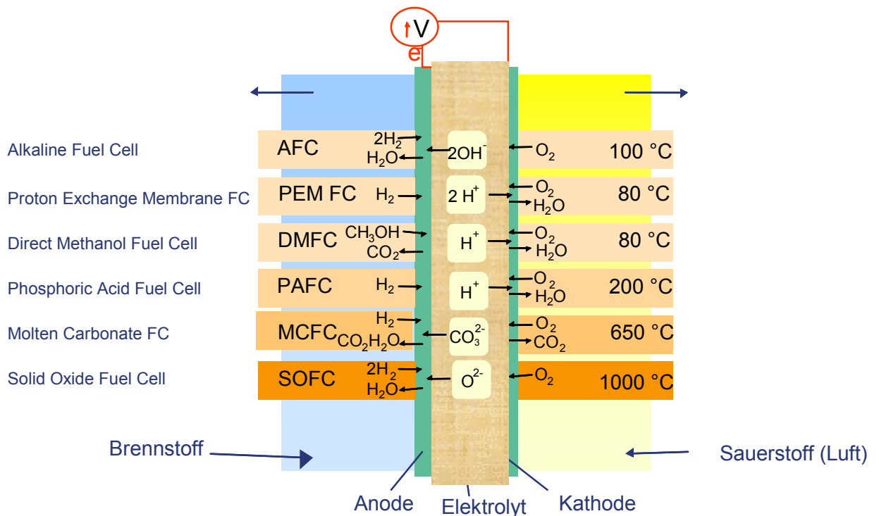
Abbildung 4-7: Funktionsprinzip von Brennstoffzellen
