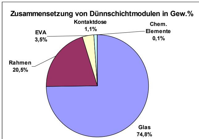
Abbildung 4-40: Zusammensetzung eines Dünnschicht PV-Moduls
