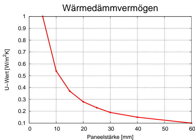
Abbildung 4-49: Wärmedämmvermögen eines Vakuum-Isolations-Paneels in Abhängigkeit der Paneelstärke
