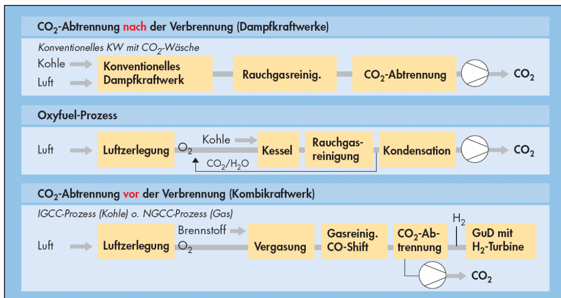
Abbildung 4-45: Schematische Darstellung der drei Carbon-Capture-Verfahren
