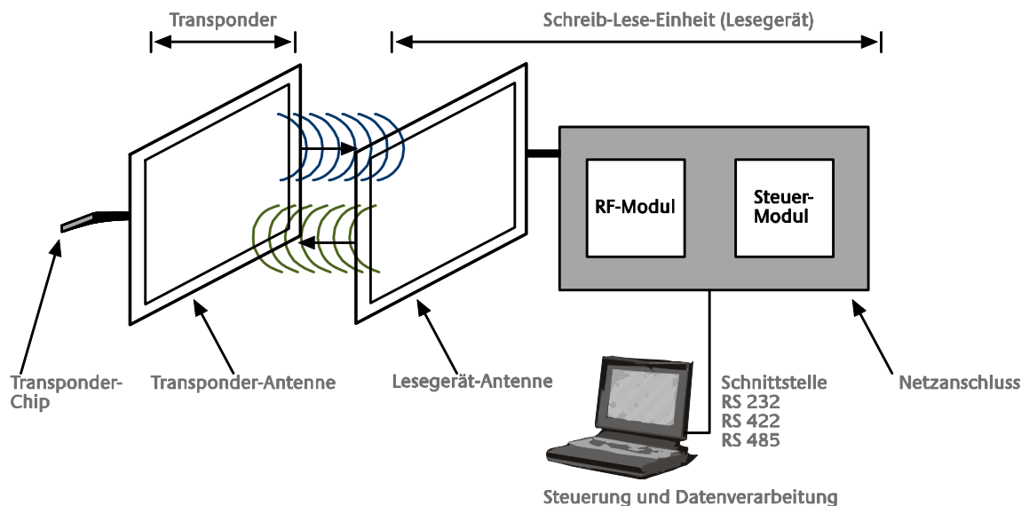
Abbildung 4-16: Schematischer Aufbau eines RFID-Systems
