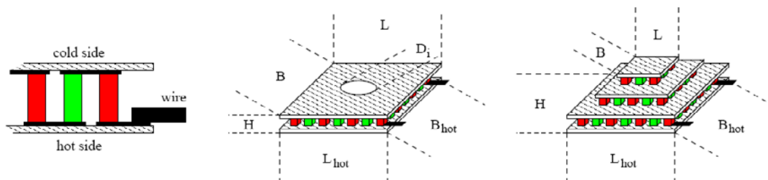
Abbildung 4-31: Schaltprinzip und Aufbau von thermoelektrischen Generatoren
