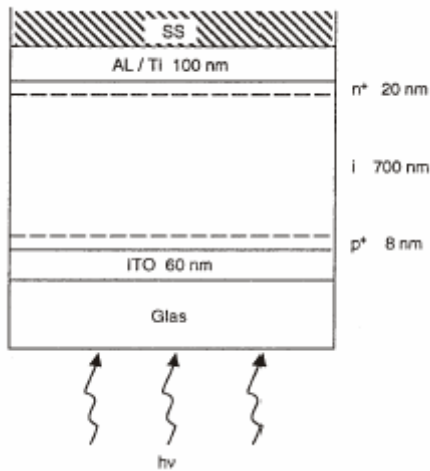
Abbildung 4-36: Aufbau einer Solarzelle aus amorphem Silizium
