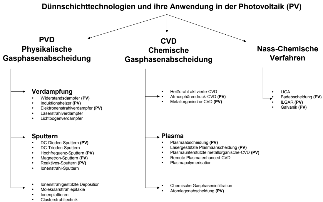
Abbildung 4-34: Überblick über die verschiedenen Dünnschichttechnologien
