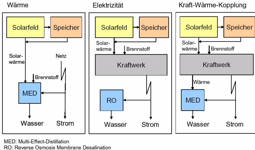
Abbildung 4-54: Meerwasserentsalzung im Systemverbund mit solarthermischen Kraftwerken
