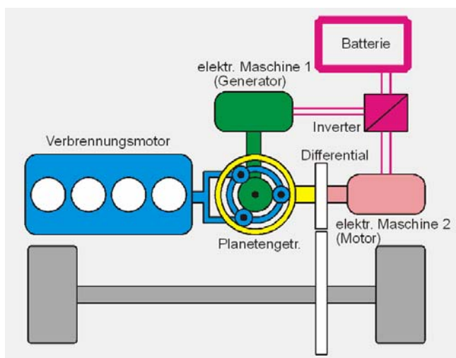
Abbildung 4-4: Baukonstruktion eines Toyota Prius mit Leistungsverzweigung
