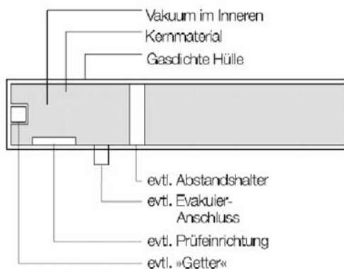
Abbildung 4-47: Schematischer Aufbau eines Vakuum-Isolations-Paneels
