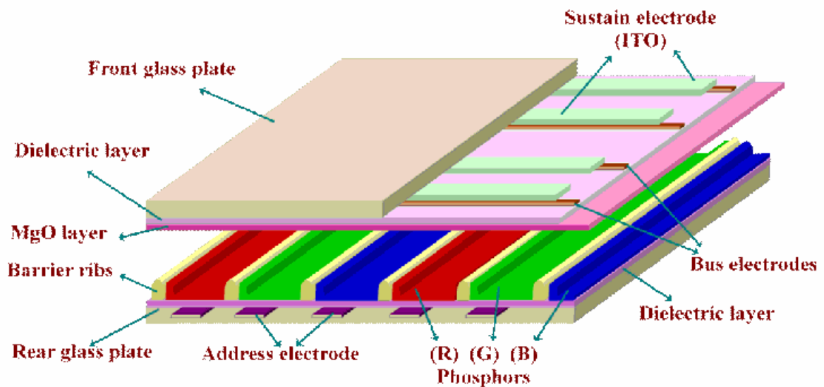
Abbildung 4-19: Schematischer Aufbau eines PDPs
