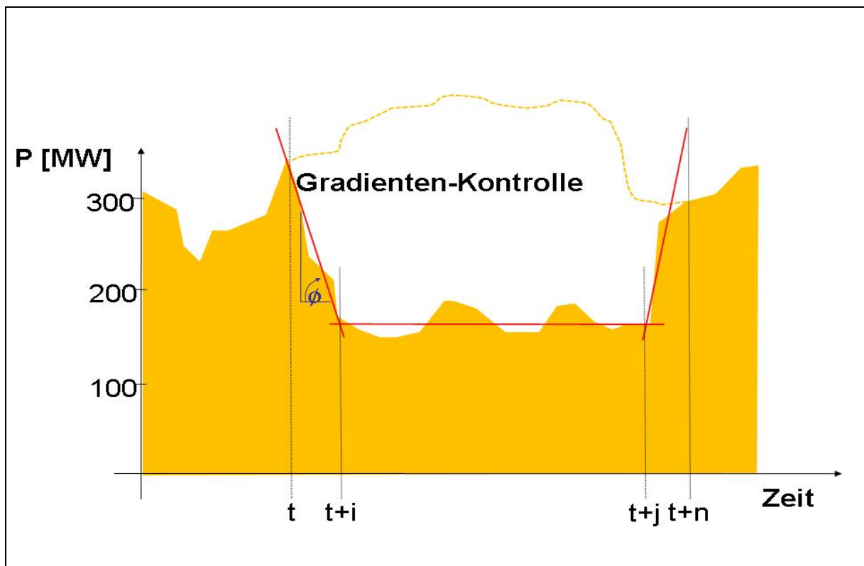
Abbildung: Wirkleistungsregelung – Gradientenkontrolle mit dem WCMS
