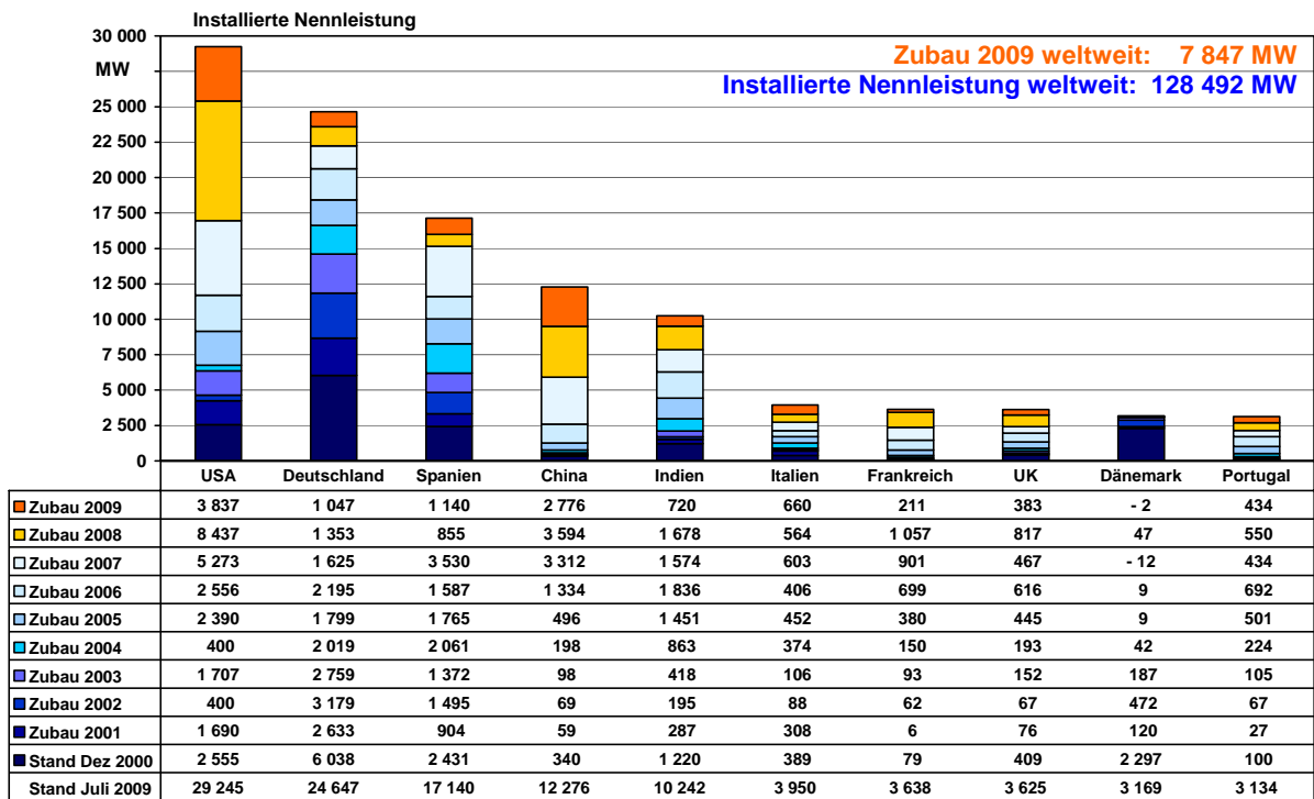
Abbildung: Weltweit installierte Windleistung
