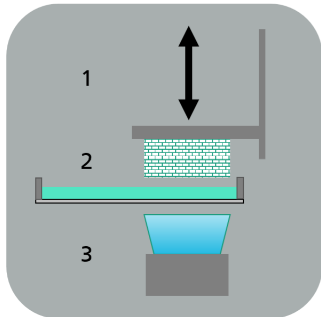
Bild 4: Schema LCM-Verfahren zur Formgebung; Baugröße: 76 \times 43 \times 150 mm 3 .
