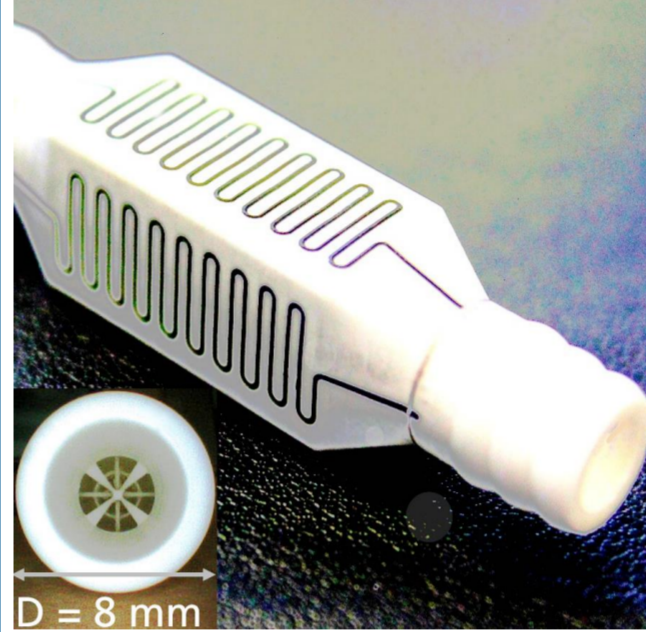
Bild 5: 3D-Fluidmischer mit Heizernetzwerk ( R = 400 \Omega ); Endoskopbild (Eingangseite); Fluidanschlüsse D = 8 mm.
