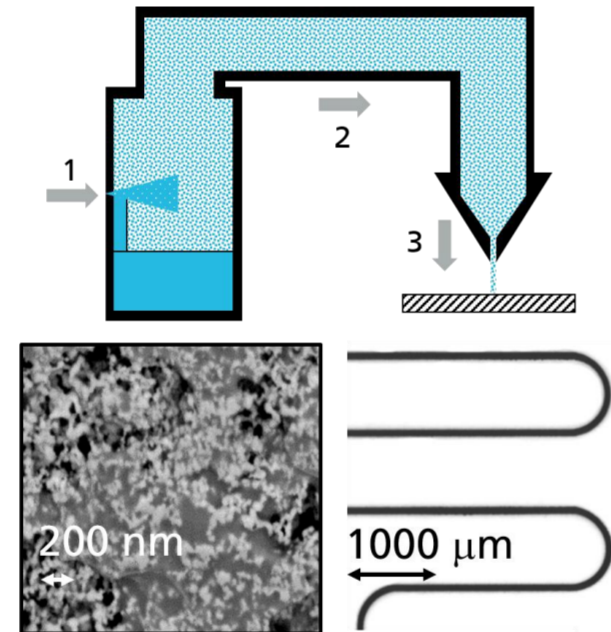
Bild 2: Schema Aerosoldruckverfahren; Leiterbahn nach dem Einbrand (Mikroskop) und FESEM-Analyse.
