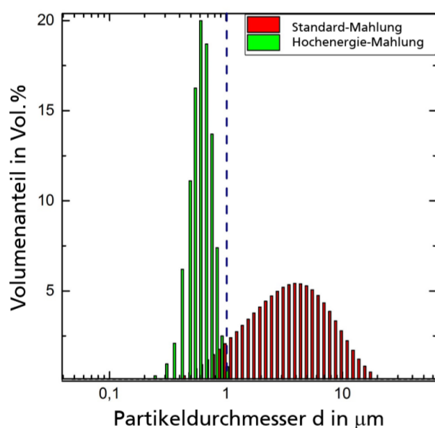
Bild 1: Partikelgrößenverteilung bei der Glasaufbereitung für Sub- \mu -Funktionstinten durch Hochenergie-Mahlung.
