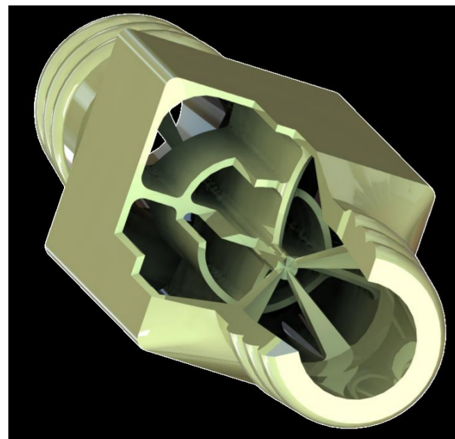
Bild 3: Konstruktionszeichnung des Fluidmischers nach Auslegung und Simulation.
