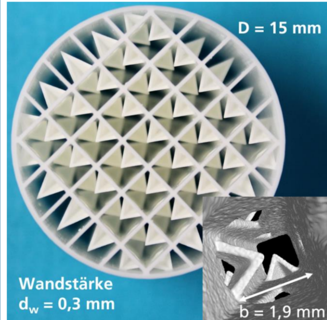
Bild 7: \text{Al}_2\text{O}_3 -Wabe mit Strömungsleiterelementen; Computertomographie (CT) der Kanalstruktur.
