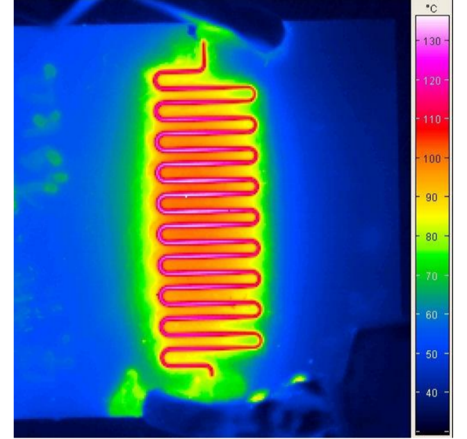
Bild 6: Temperaturmessung mit einer Wärmebildkamera am konform temperierten Fluidmischer ( \theta_{\max} > 130 °C).
