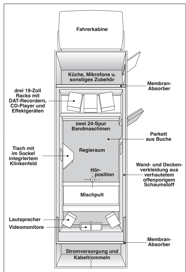
Bild 1: Blick von oben in den Übertragungswagen
