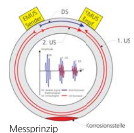
Messprinzip
