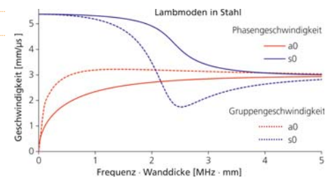
Dispersionsdiagramm von Lambwellen
